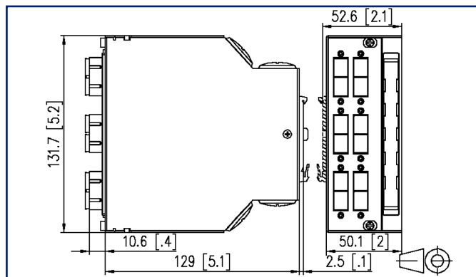
Schéma dimensionnel
