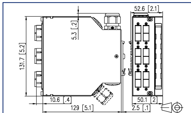
Schéma dimensionnel
