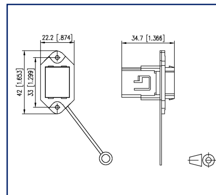
Schéma dimensionnel
