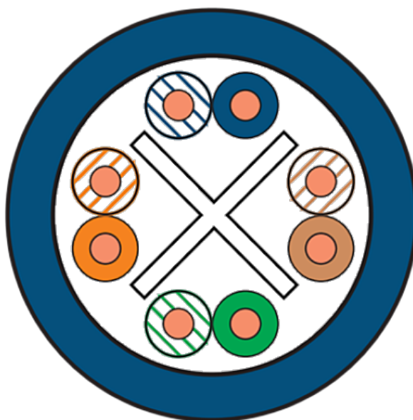
Cat.6 Übertragungseigenschaften bei 20°C (Nominal)
