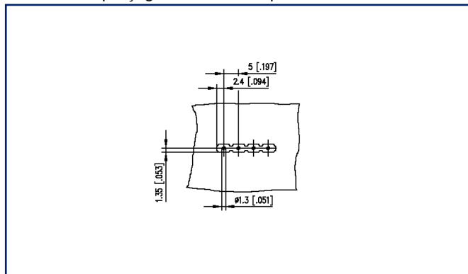
Schéma de perçage à titre d'exemple
