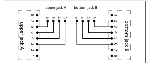
Schaltbild 130886-0203-E Connection Diagram 130886-0203-E
