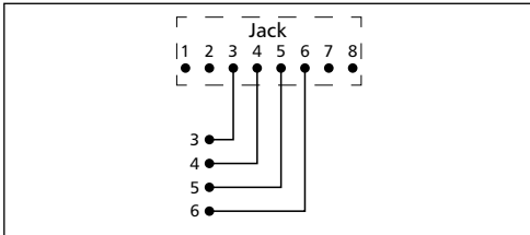
Schaltbild 130814-0203-E Connection Diagram 130814-0203-E
