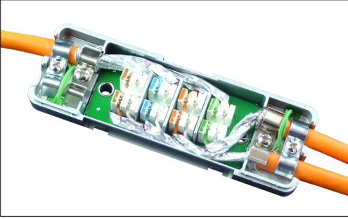
Kabelaufteilung 1x8 auf 2x4. Ggf. von der Kabelkonfektion (siehe Bild Kabelkonfektion Variante 1 und Variante 2) abweichende Adernpaar- und Schirmmlängen beachten. Cable splitting 1x8 to 2x4. Respect if necessary different lengths for wire pairs and shield foil (see fig. cable preparation variant 1 and variant 2).
