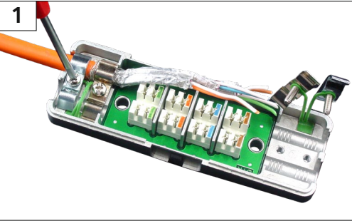
Zugentlastung und Schirmschluss anbringen. Hinweis: Für eine optimale Übertragungstechnische Performance muß der Paarschirm direkt bis zum LSA-Klemmkontakt geführt werden. Connect strain relief and shield connection. Note: To obtain the optimum of transmission performance lead the pair shield directly up to the respective LSA terminal contact.
