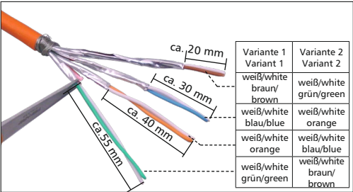
Variante 1: Kabelkonfektion mit Adernpaar weiß/braun beginnend. Variante 2: Kabelkonfektion mit Adernpaar weiß/grün beginnend.
