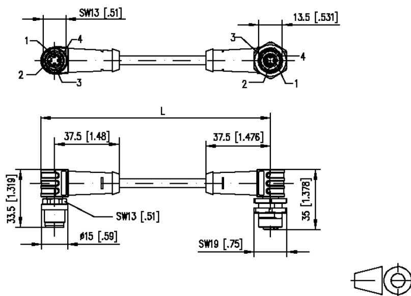
M12 jack
