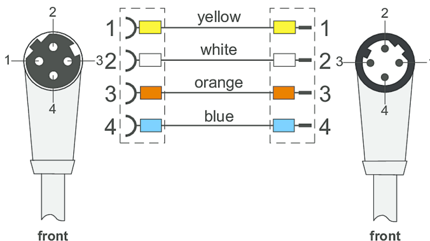
M12 jack
