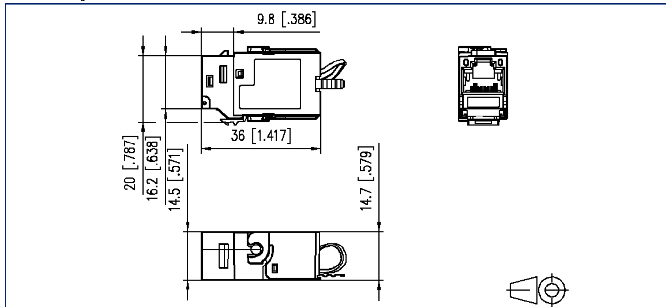
Maßzeichnung
