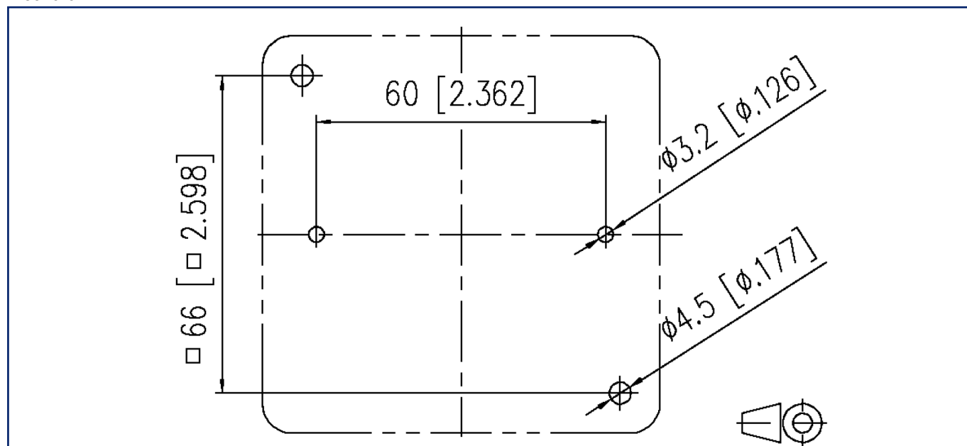
Lochbild
