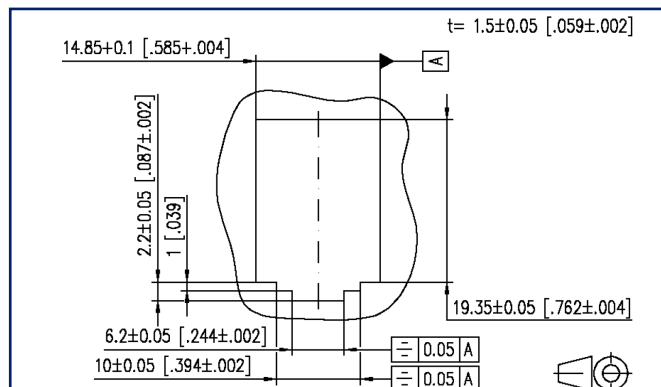
Einbauausschnitt
