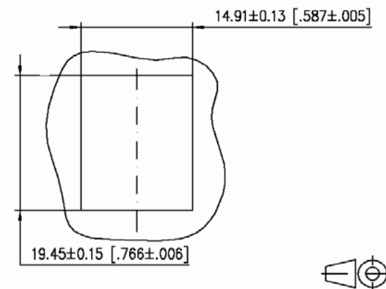
Masszeichnung Keystone
