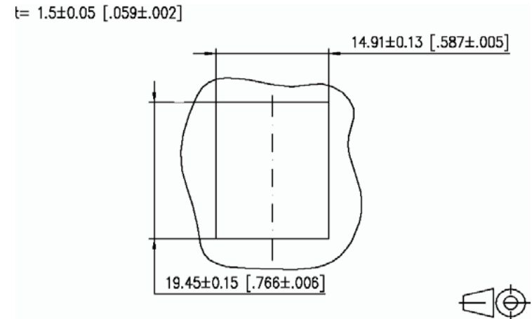
Masszeichnung Keystone
