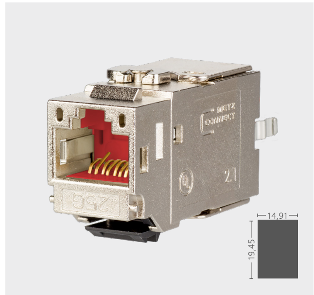
25Gmodul K
