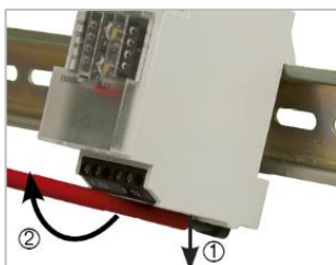
Abbildung 2 Demontage des MR-GW
