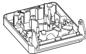
Sockelteil mit integrierter Faserführung Base part with integrated fiber guiding Socle avec guidage intégré de la fibre
